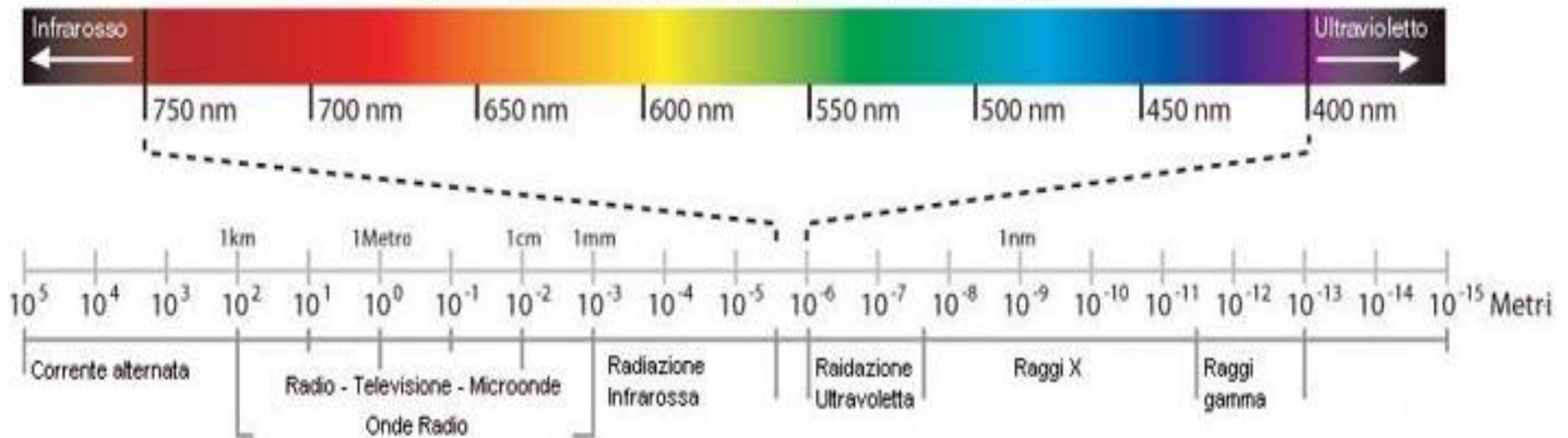
Spettro di luce visibile all'occhio umano
